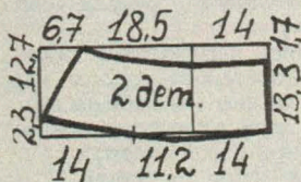
МОДЕЛЬ 3: кокетка переднего полотнища юбки.
