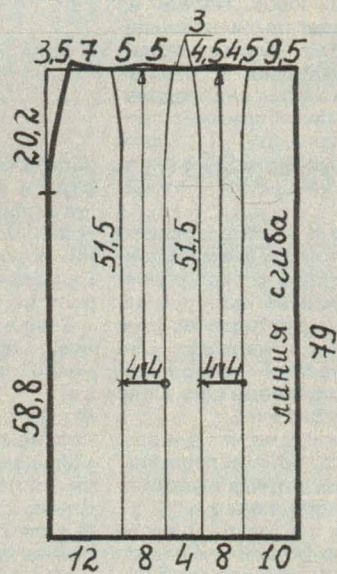
МОДЕЛЬ 2: переднее и заднее полотнища юбки (2 дет.).
